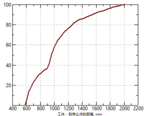
横向焊合（接棒长度）与实际对比
