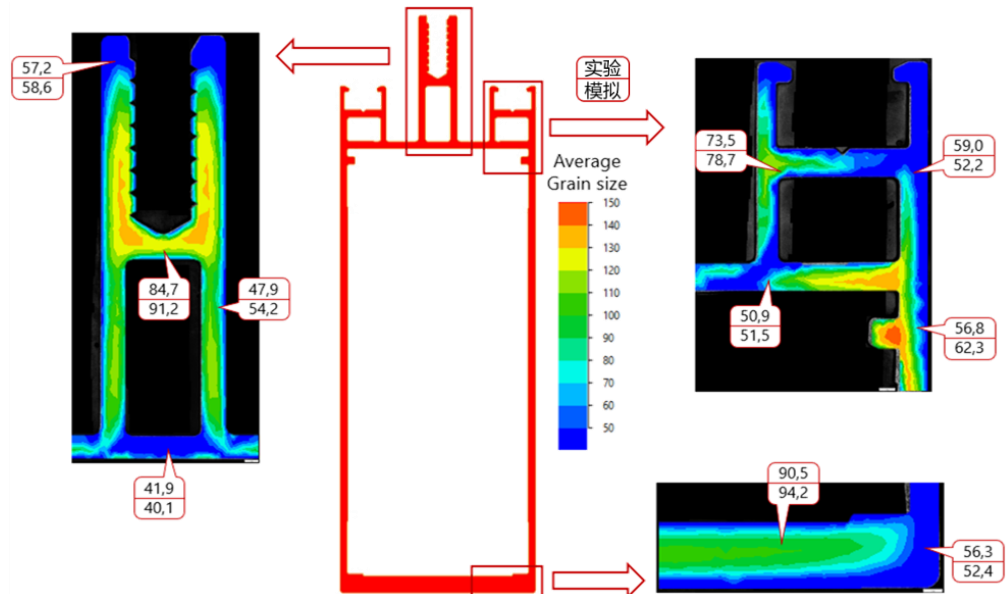
实验与模拟晶粒尺寸对比
