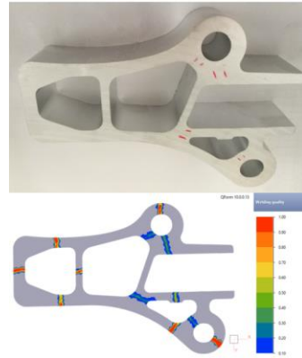
焊合质量分析（通过焊合位置的颜色判定）
