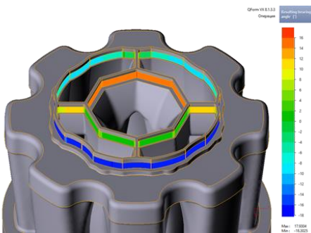
工作带偏斜角度
