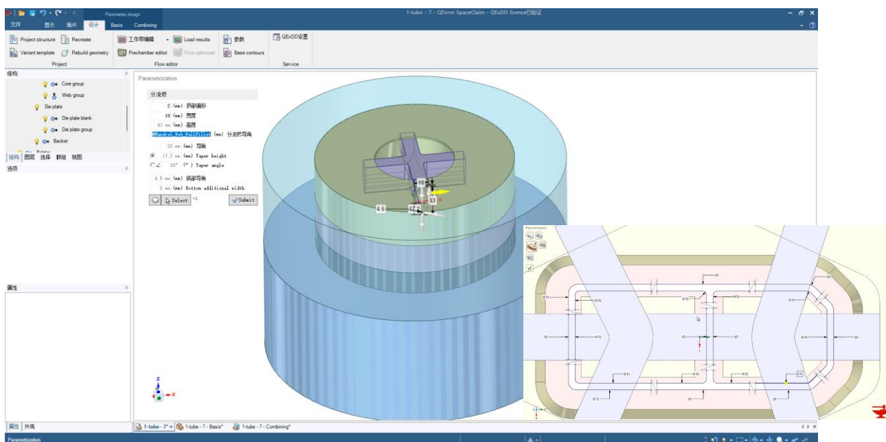
QExDD 界面 (分流桥参数设置、工作带调整)
