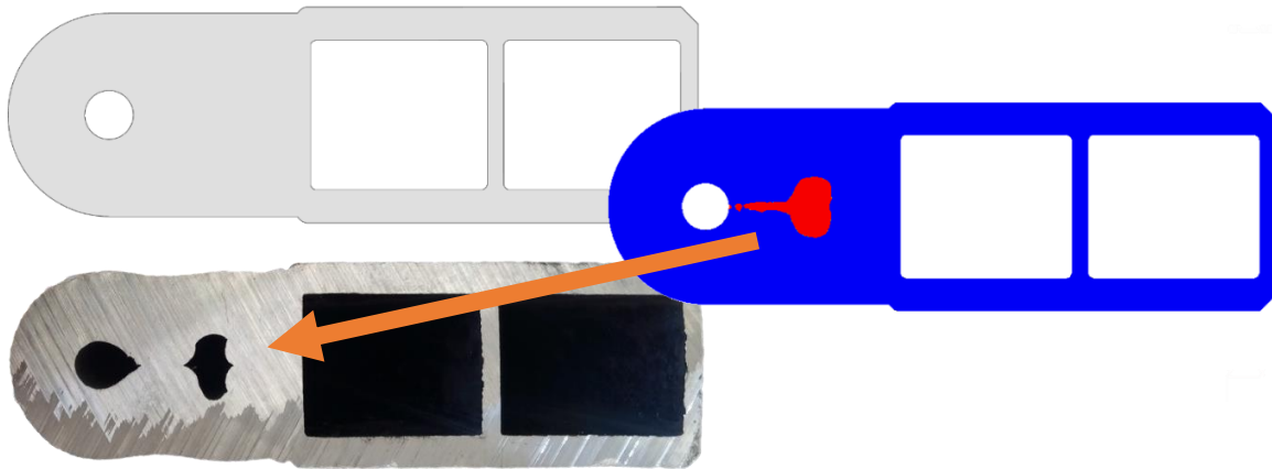
皮下缩尾和中心缩尾分析
