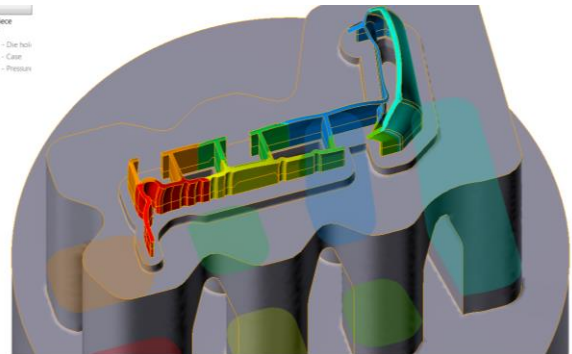
焊合线位置模拟结果（不同颜色交接处）
