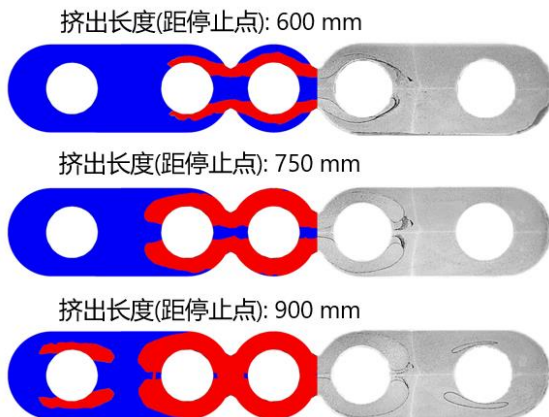
横向焊合（接棒长度）与实际对比
