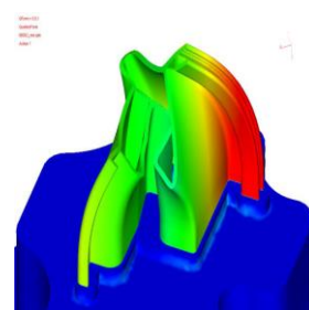
料头形状和速度场分布
