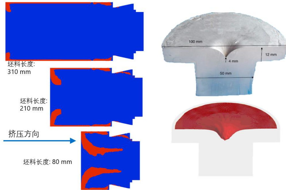
皮下缩尾和中心缩尾分析
