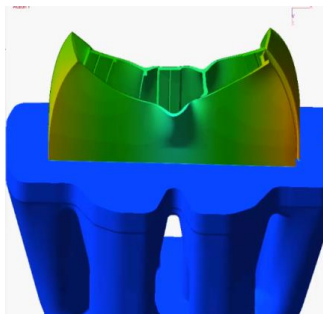
分流模 型材料头
